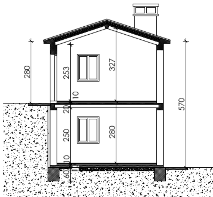
PRESJEK A-A 1:100
