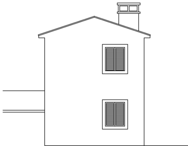
ISTOČNA FASADA 1:100
